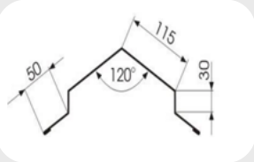
Driehoek nok
