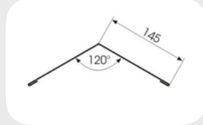
Platte nok
