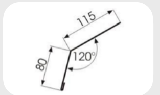
Onderlegger
